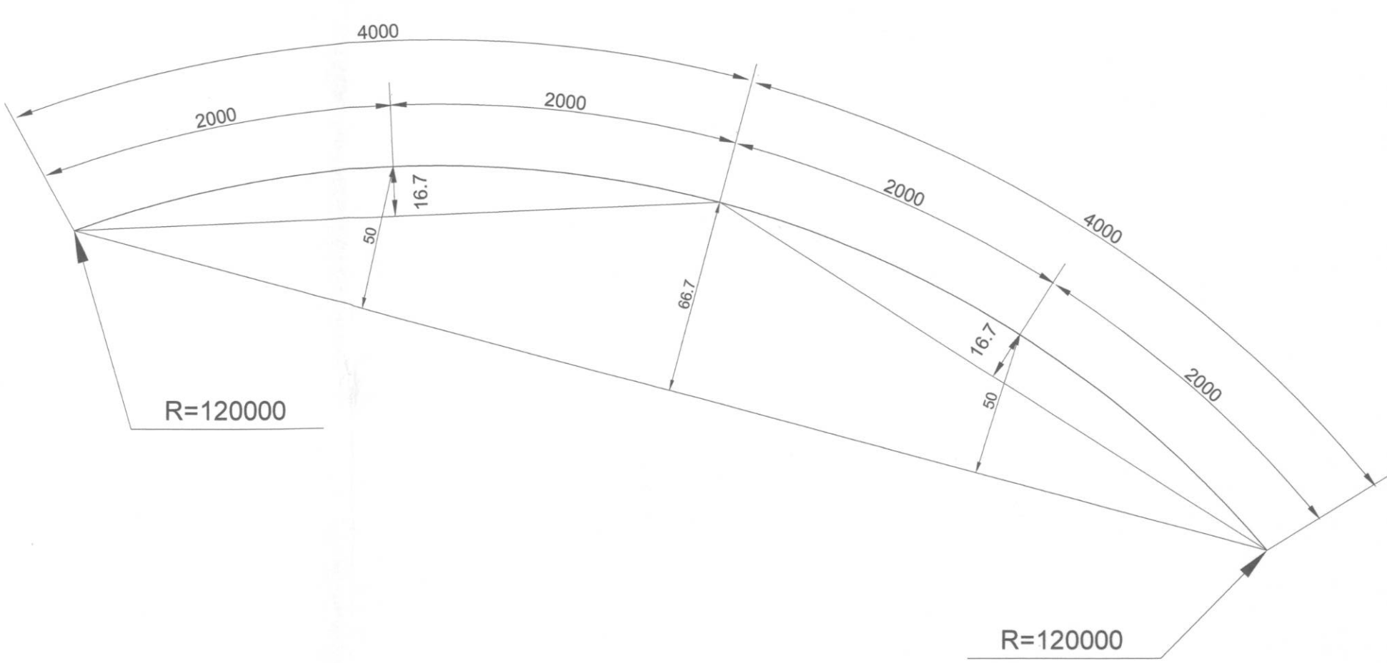
ESQUEMA DEL CURVAMIENTO DE LA AGUJA (L=8000) SOBRE FILA DIRECTRIZ
