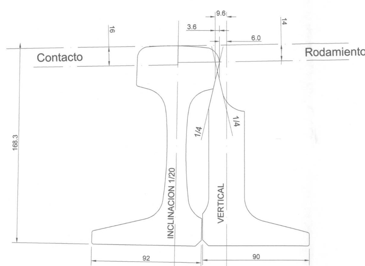
SECCION A-A'
