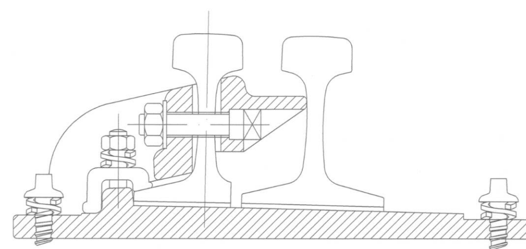
CORTE A-A S/E
