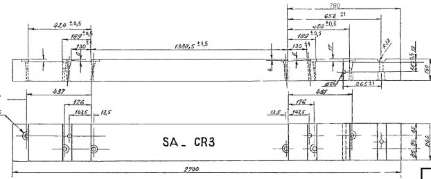
3 ème traverse de crosselette alimentation en alignement marquée SA CR3
