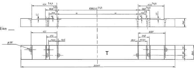
1 ère traverse de crosselette alimentation en alignement marquée SA CR1
