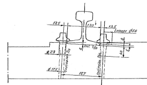
COUPE AU DROIT D'UN RAIL échelle : 1/2
