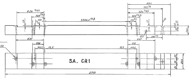
1 ère traverse de crosselette alimentation en alignement marquée SA CR1
