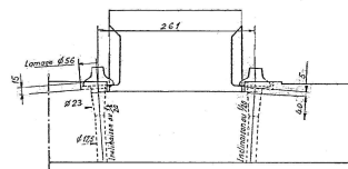
COUPE AU DROIT D'UNE PIÈCE DE ROULEMENT échelle : 0,5g
