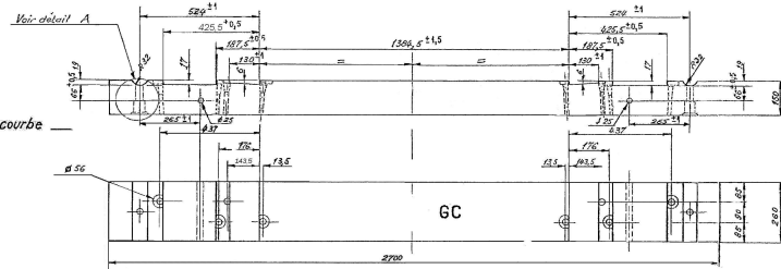
COUPE AU DROIT D'UNE PIÈCE DE ROULEMENT échelle : 0,5g
