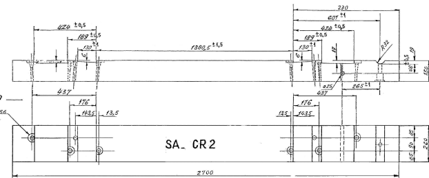
2 ème traverse de crosselette alimentation en alignement marquée SA CR2
