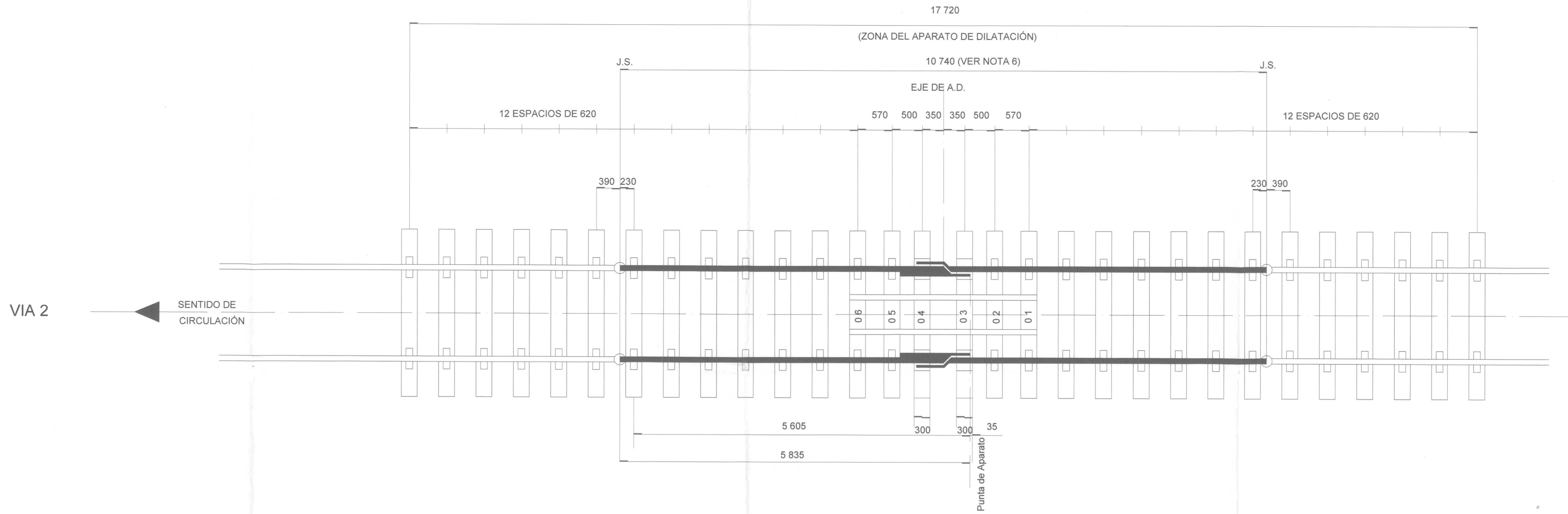
ZONA DE APARATO DE DILATACIÓN VÍA 2 S/E
