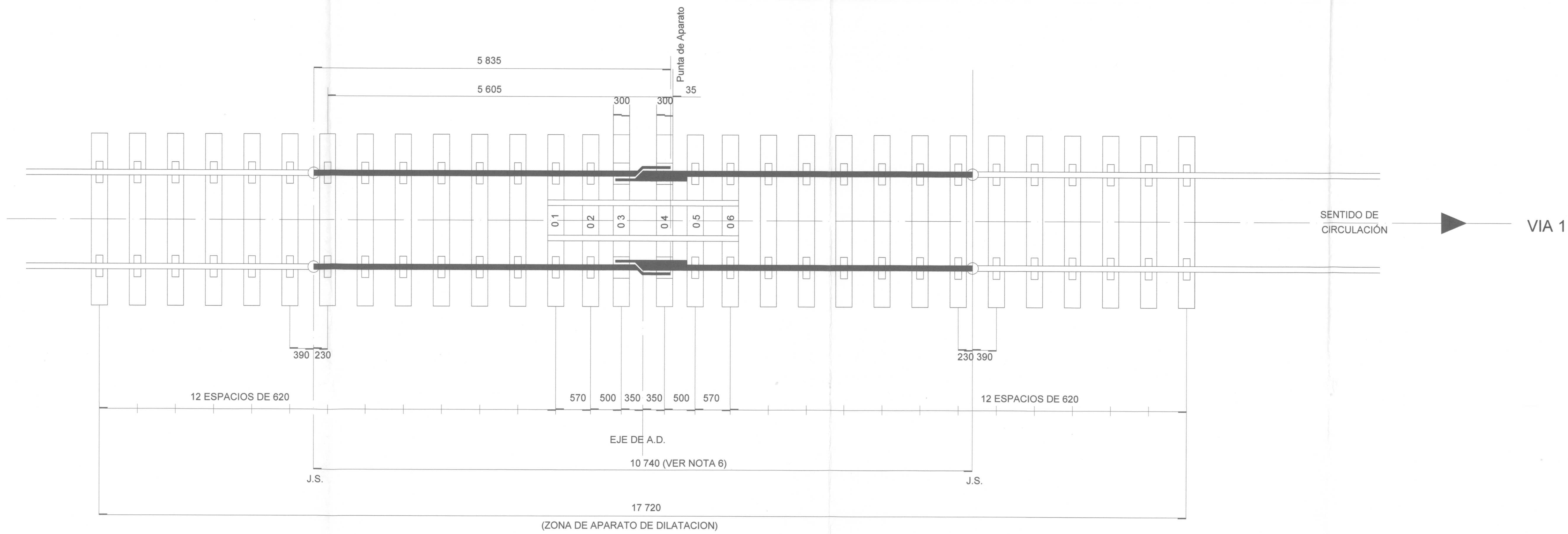
ZONA DE APARATO DE DILATACIÓN VÍA 1 S/E
