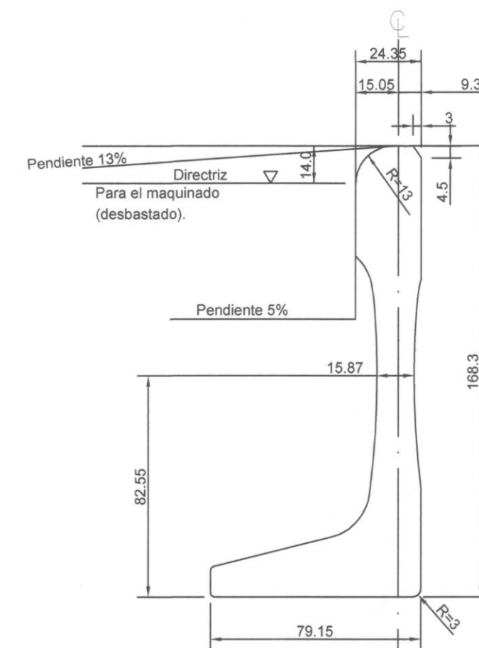
SECCION B-B ESCALA 1:2
