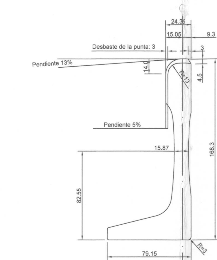
VISTA A ESCALA 1:2
