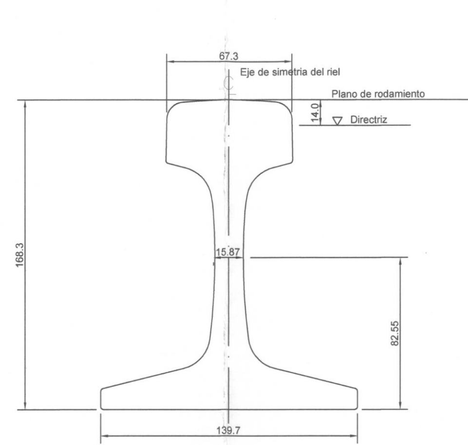
SECCION DEL RIEL 115 RE ESCALA 1:2
