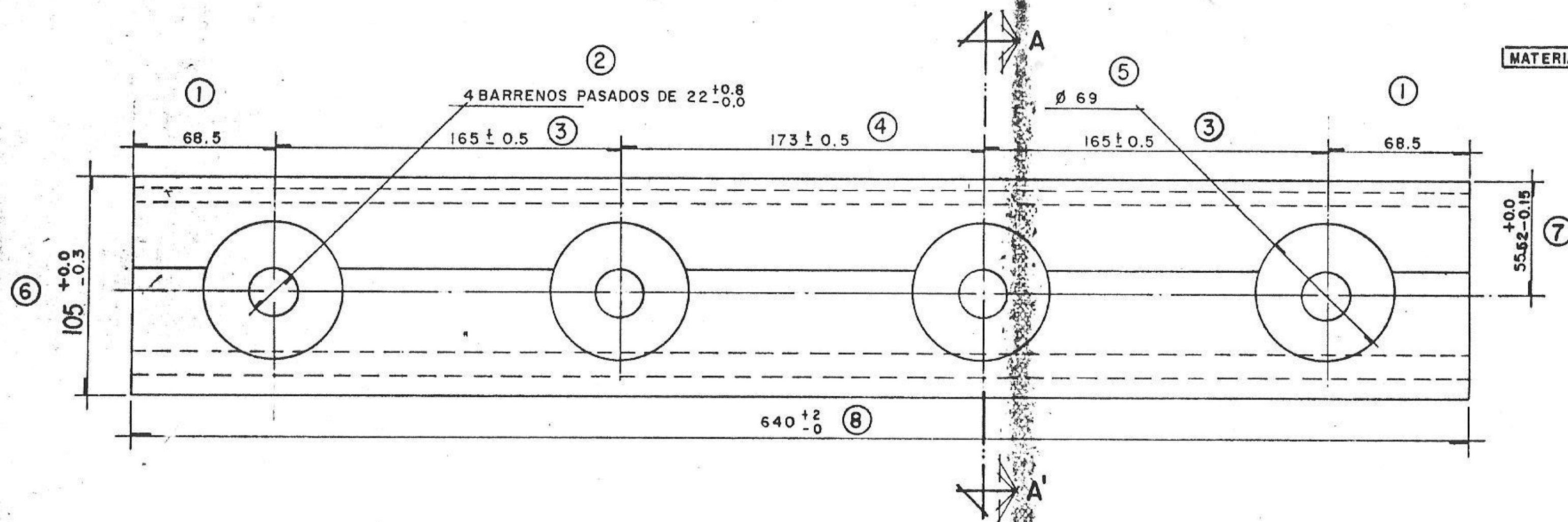
PLANTA
